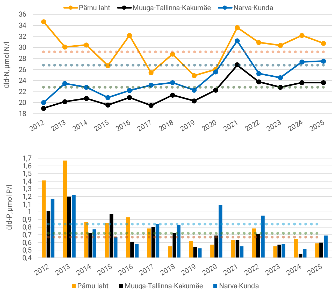
Joonis 10. Üldlämmastiku (üld-N, µmol N/l) ja -fosfori (üld-P, µmol P/l) aasta keskmiste kontsentratsioonide trend kolmes rannikumere püsiseirekogumis. Katkendlike joontega on näidatud ka "hea" ja "kesise" klassi piiride läviväärtus kõigis kolmes kogumis.
