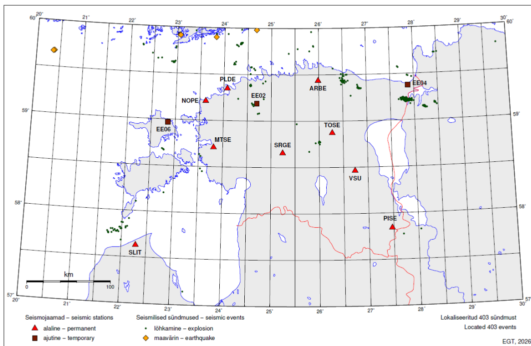
Joonis 14. Eesti geoloogiateenistuse poolt 2025. a seismilise seire raames lokaliseeritud sündmused. Punased kolmnurgad: alalised seismojaamad; pruunid nelinurgad: ajutised jaamad; rohelised täpid: tehnogeensed sündmused; oranžid rombid: maavärinad.
