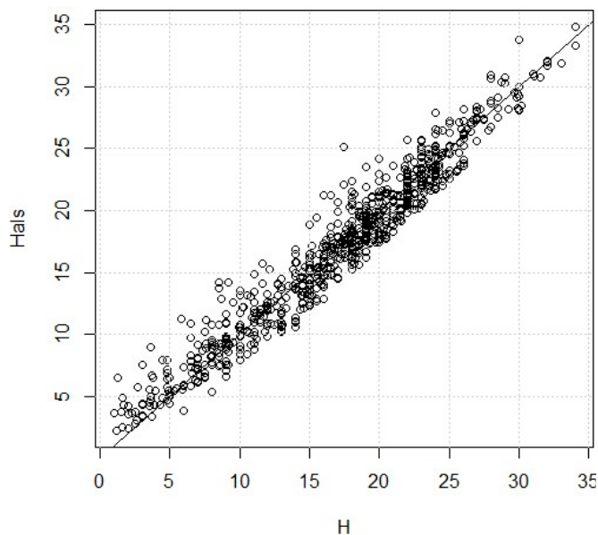
Joonis 7. Edela-Eesti SMI proovitükkidel inventeeritud kõrguse (H) ja SW 2023 mudeliga arvatud kõrguse ( H_{ALS} ) korrelatsioon (m); lisatud 1:1 joon
