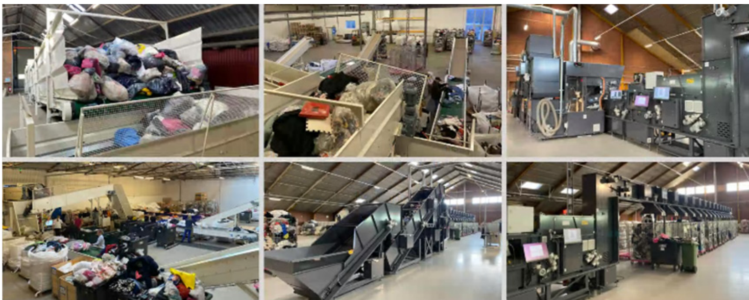
Foto 1. NewRetex täisautomaatne sortimisliin. Allikas: kuvatõmmis NewRetex tehnoloogia ettekandest, 2024.
