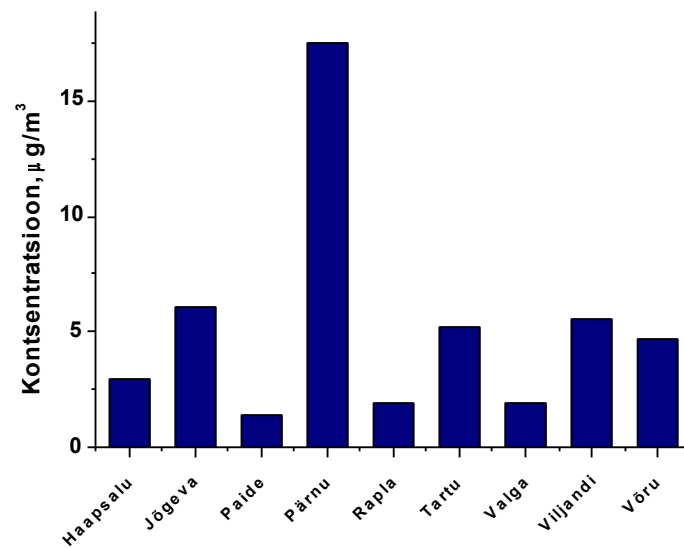
Joonis 13 SO 2 maksimaalne 1h kontsentratsioon
