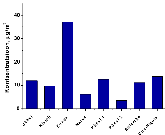
Joonis 4 SO 2 maksimaalne 24h kontsentratsioon
