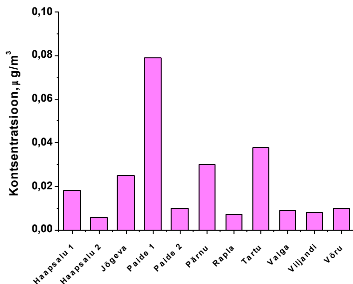
Joonis 22 Pb perioodi keskmine kontsentratsioon
