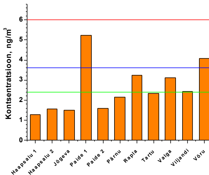
Joonis 19 As perioodi keskmine kontsentratsioon
