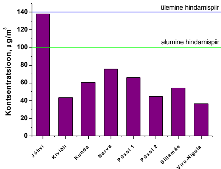
Joonis 5 NO 2 maksimaalne 1h kontsentratsioon
