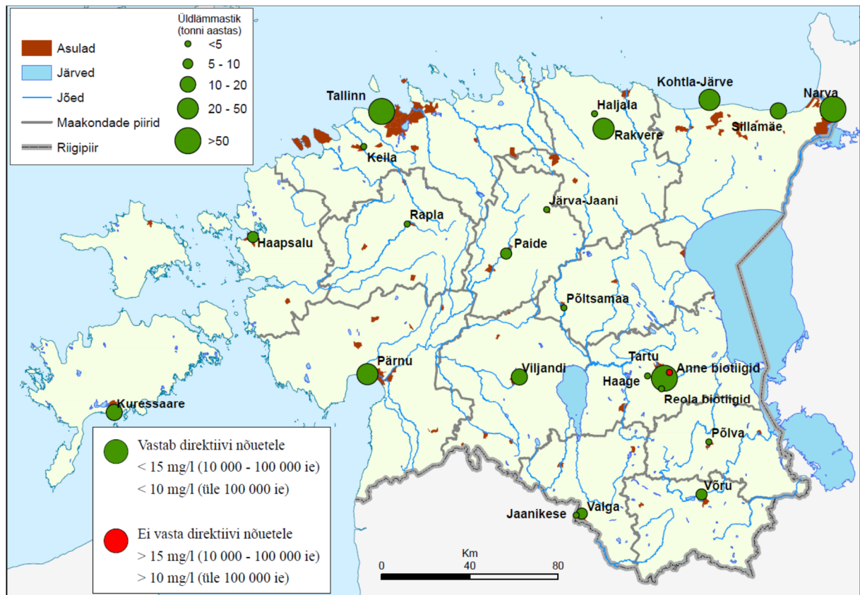
Joonis 6. Üle 10 000 ie reoveekogumisalade reostuskoormus ja lämmastiku vastavus direktiivi nõuetele aastal 2012
