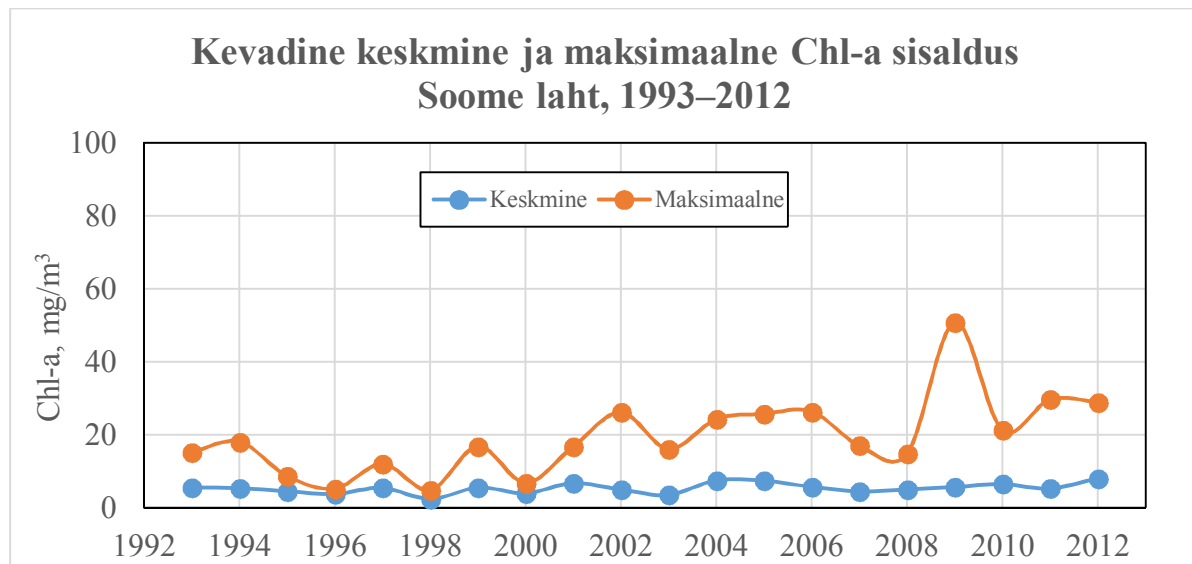
Joonis 20. Kevadised klorofüll-i sisaldused Soome lahes
