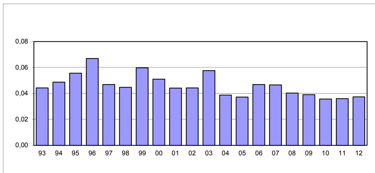
Joonis 16. Vortsjärve 1993.–2012. aasta keskmised P üld sisaldused, mgP/l
