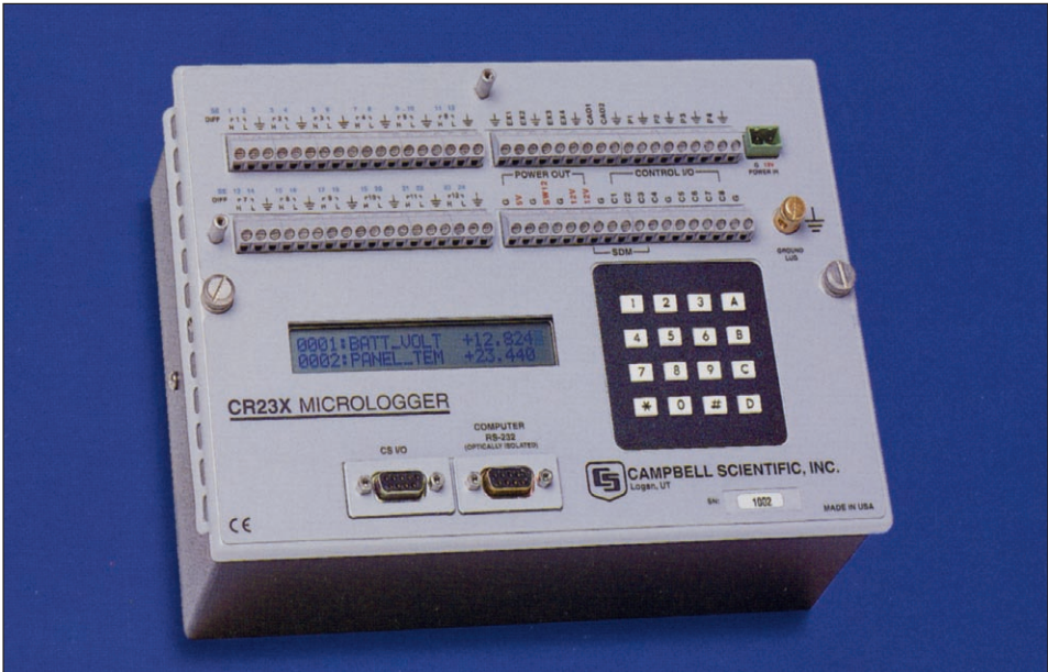
Fig. L.4.2.2-1. Campbell Scientific datalogger CR23X.
