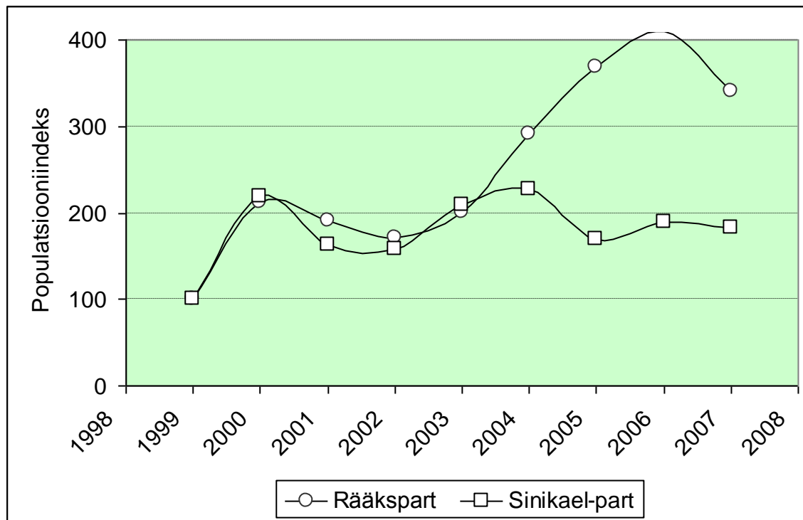
Joonis 4. Rääks- ja sinikael-pardi pesitsusaegse arvukuse muutused Lääne-Eesti rannaniitudel aastail 1999-2007. Populatsiooniindeksi väärtus 1999.a. on 100.
