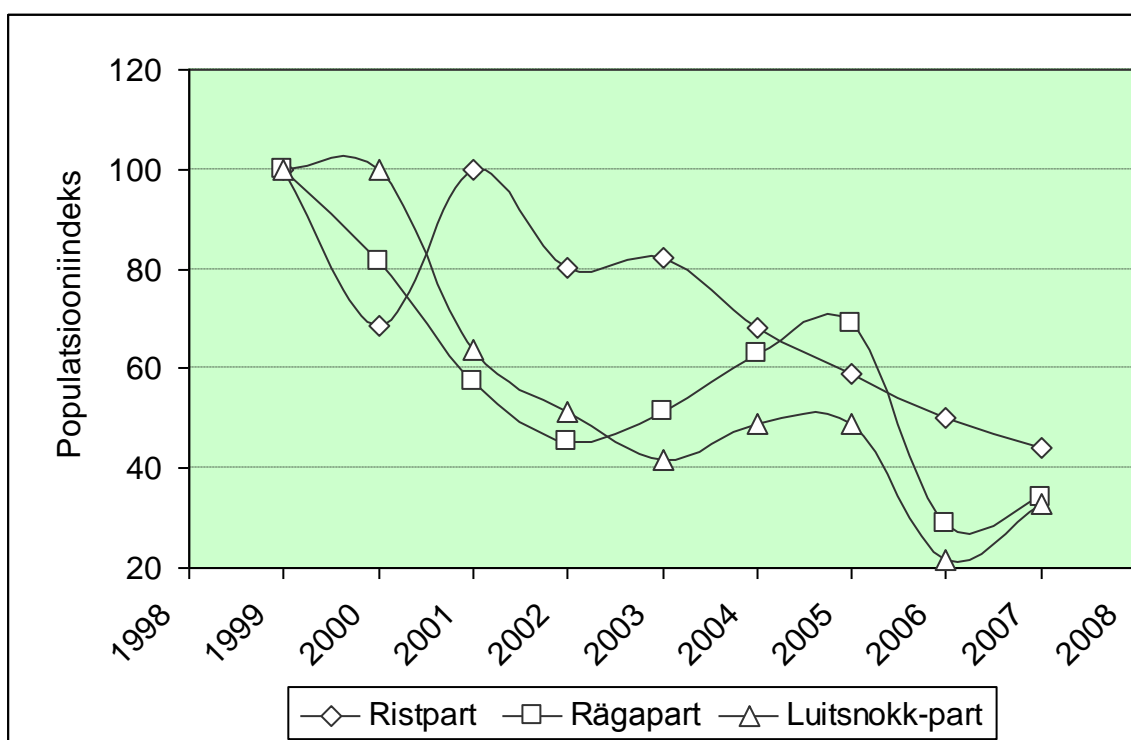
Joonis 3. Rist-, räga- ja luitsnokk-pardi pesitsusaegse arvukuse muutused Lääne-Eesti rannaniitudel aastail 1999-2007. Populatsioonindeksi väärtus 1999.a. on 100.
